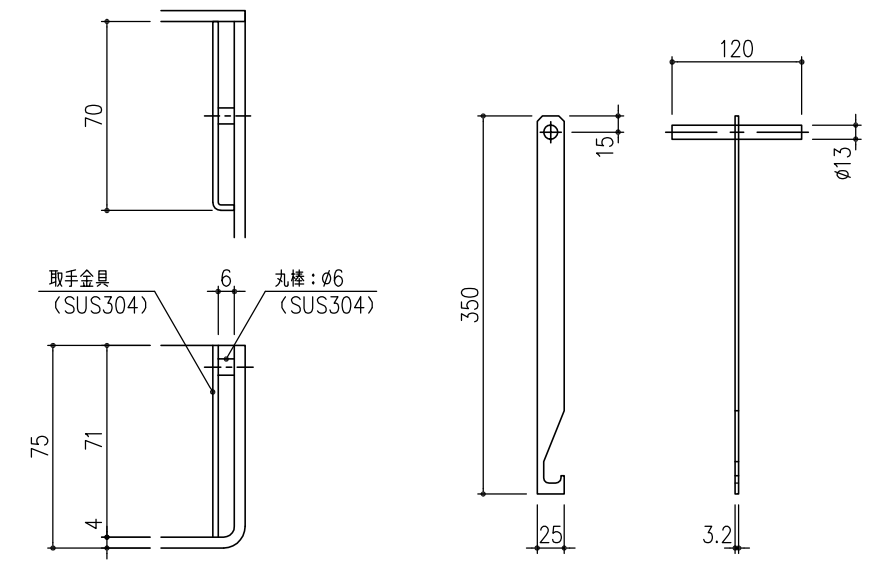
取手金具 詳細図 S=1/2 オプション：開閉フック (MF-62) (S45C) 電気亜鉛めっき
