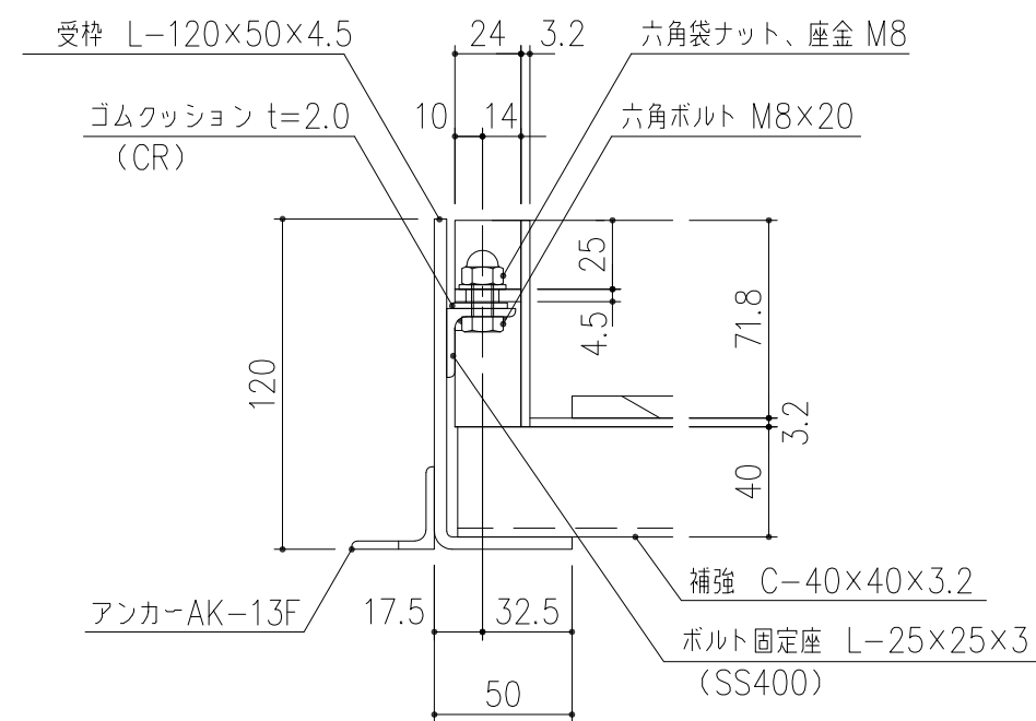
B部 詳細図 S=1/3
