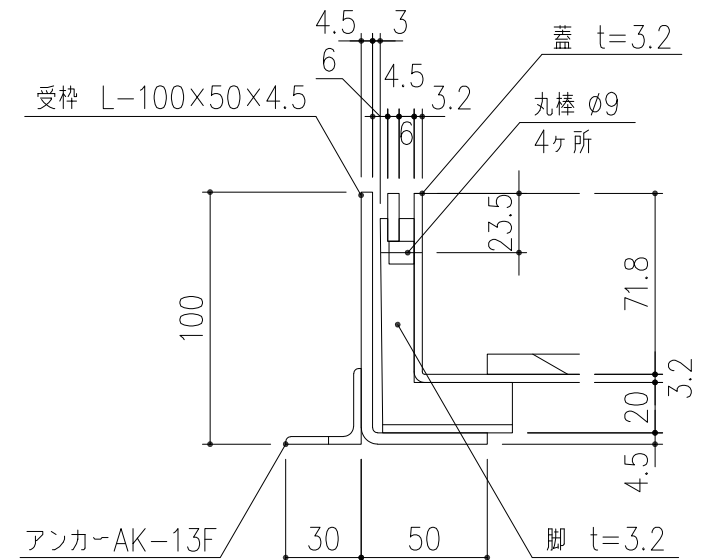
A部 詳細図 S=1/3
