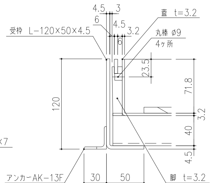
A部 詳細図 S=1/3
