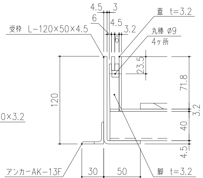
A部 詳細図 S=1/3
