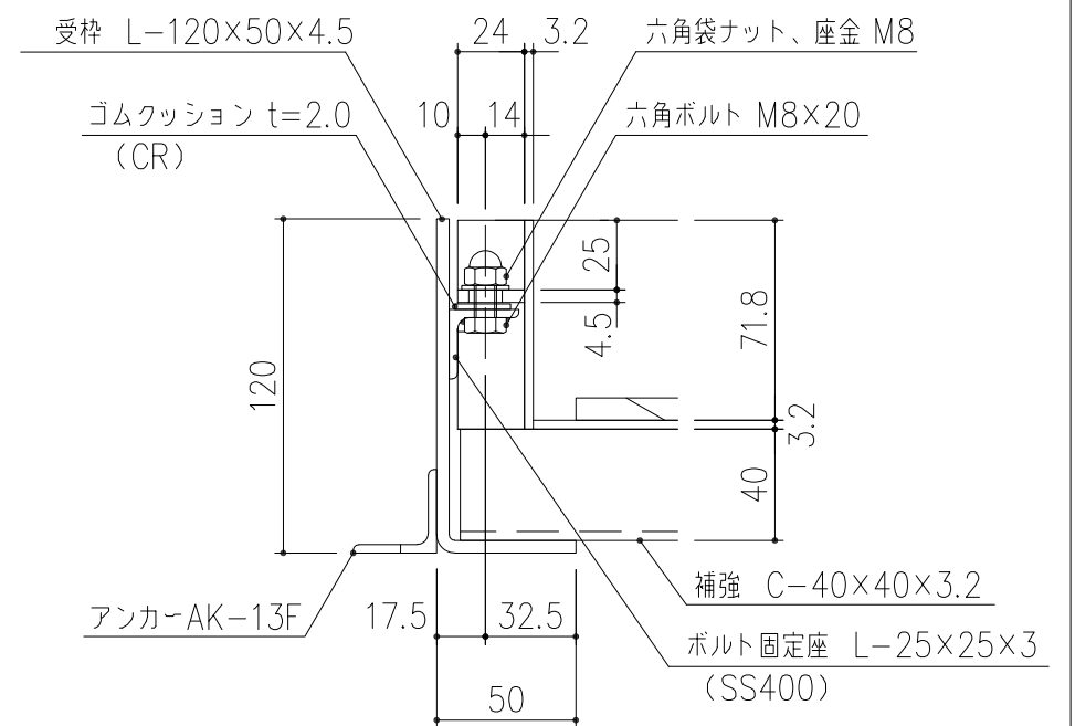
B部 詳細図 S=1/3
