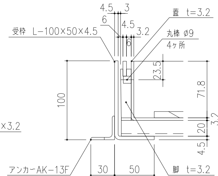
A部 詳細図 S=1/3
