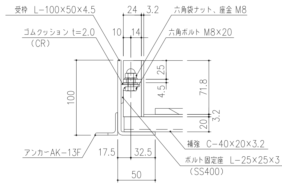
B部 詳細図 S=1/3
