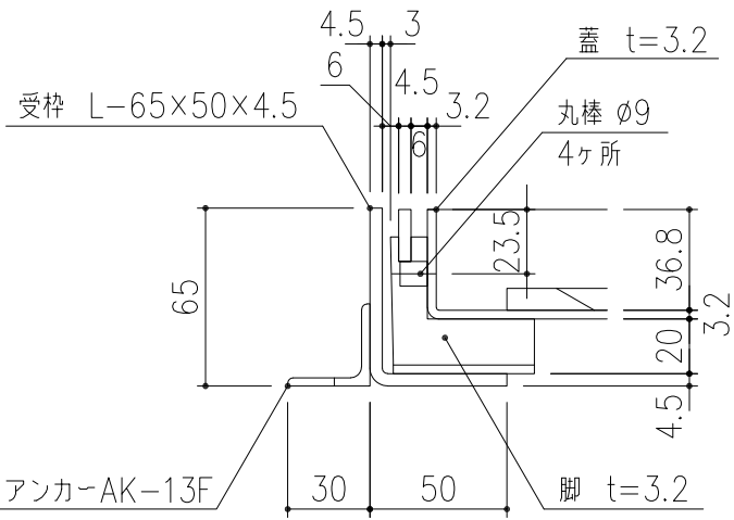
A部 詳細図 S=1/3
