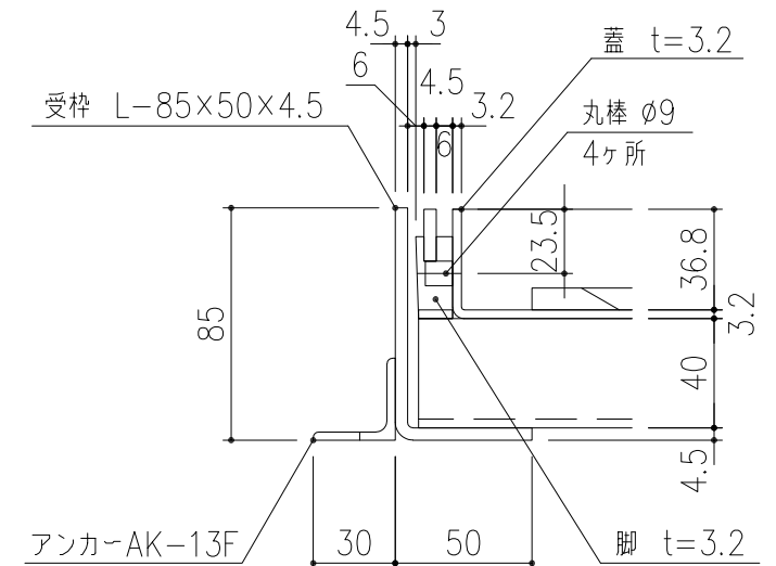
A部 詳細図 S=1/3
