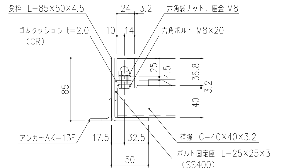
B部 詳細図 S=1/3
