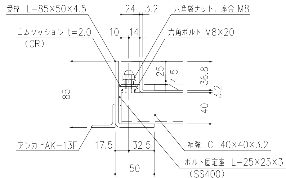
B部 詳細図 S=1/3
