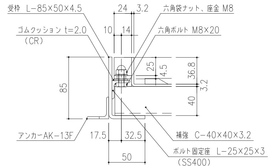
B部 詳細図 S=1/3
