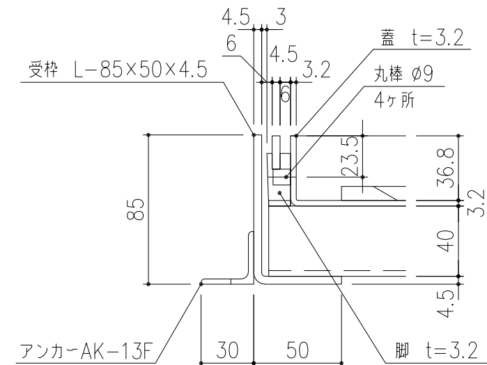
A部 詳細図 S=1/3
