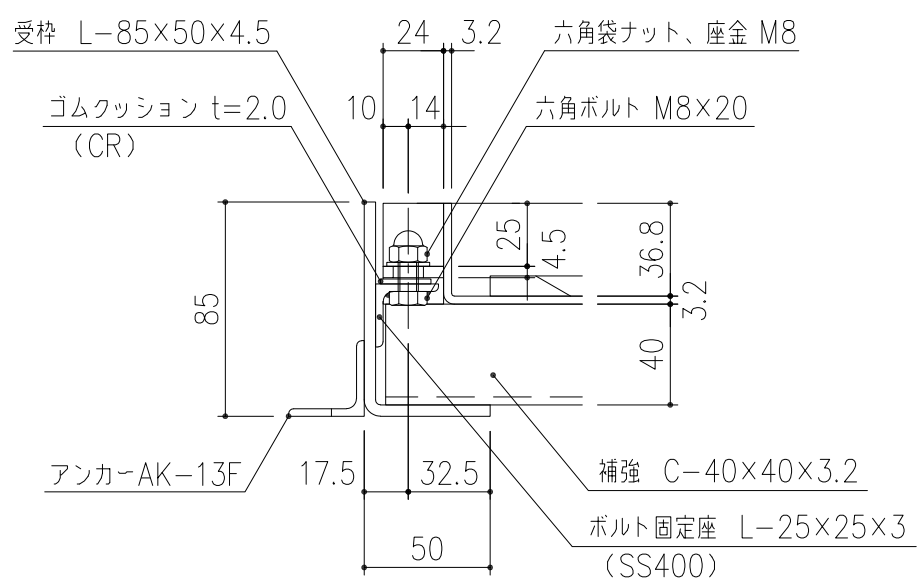
B部 詳細図 S=1/3
