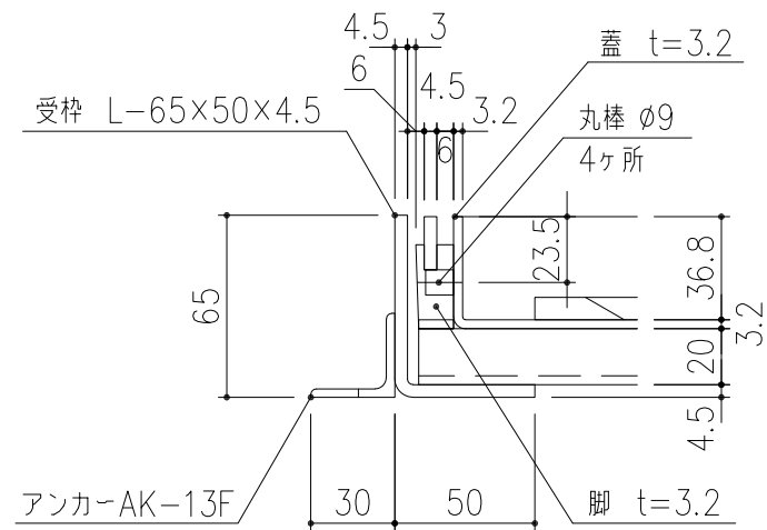
A部 詳細図 S=1/3
