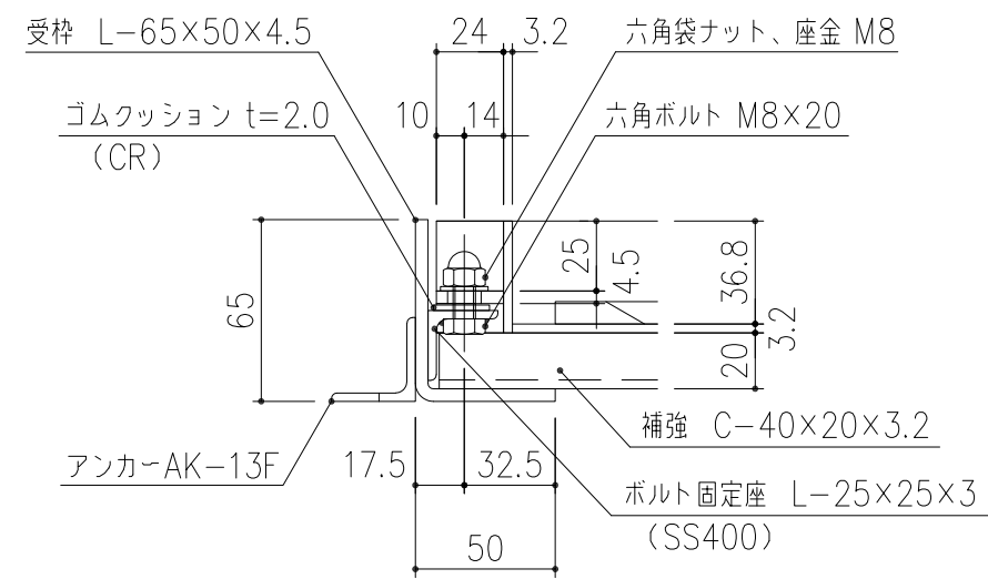
B部 詳細図 S=1/3
