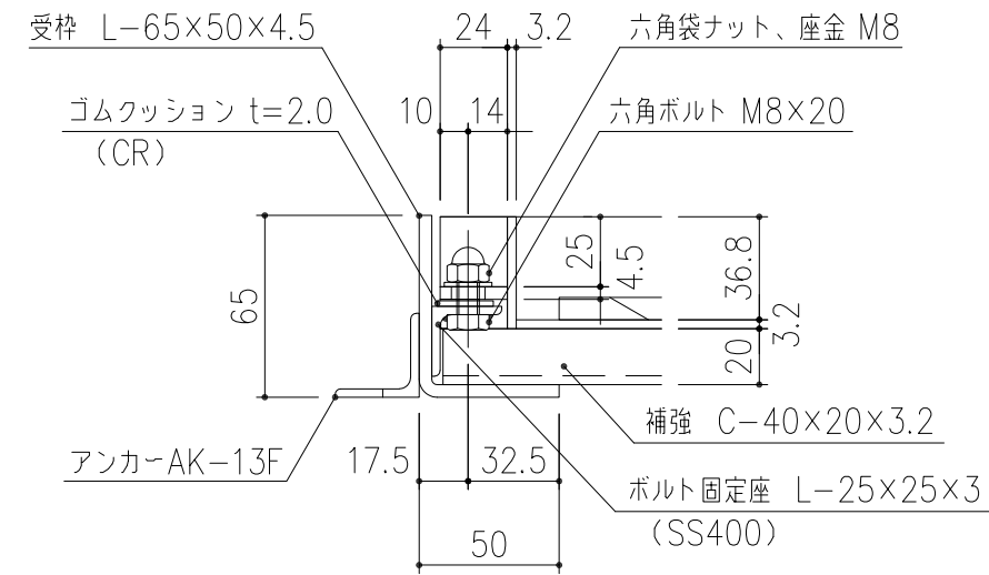
B部 詳細図 S=1/3
