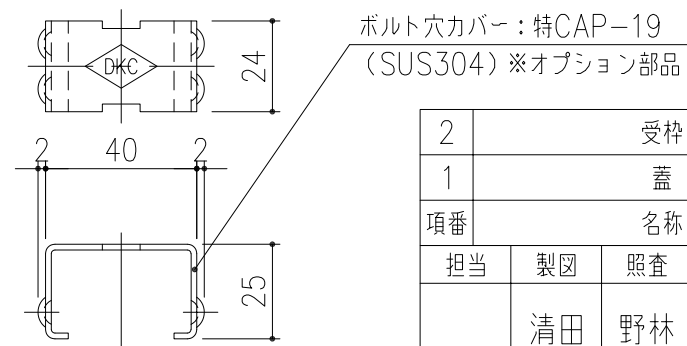
ボルト穴カバー：(特)CAP-19 詳細図 S=1/2 ※オプション部品
