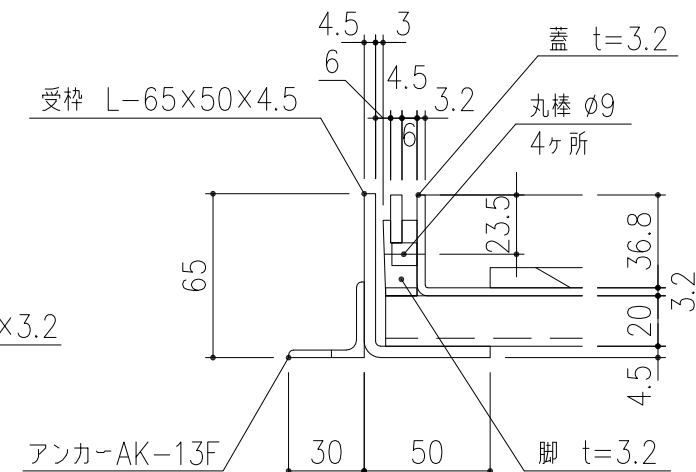
A部 詳細図 S=1/3
