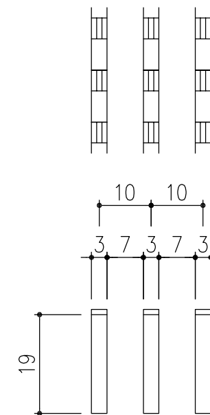
メンバー詳細図 S=1/1
