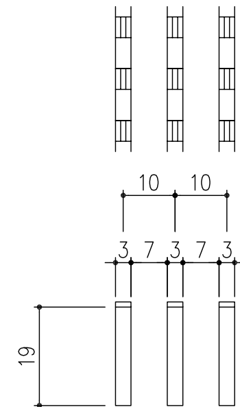
メンバーピッチ詳細図 S=1/1
