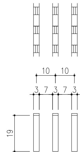
メンバー詳細図 S=1/1
