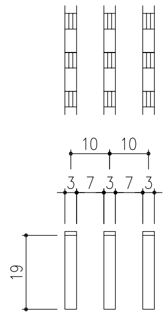
メインバー詳細図 S=1/1
