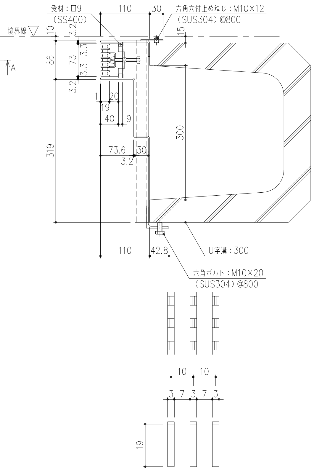
メインバー詳細図 S=1/1
