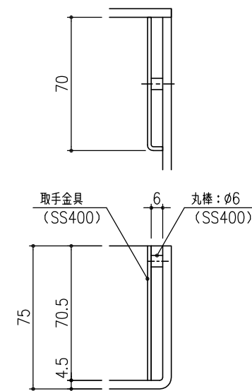
取手金具 詳細図 S=1/2
