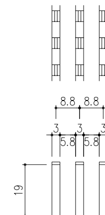
メンバー詳細図 S=1/1
