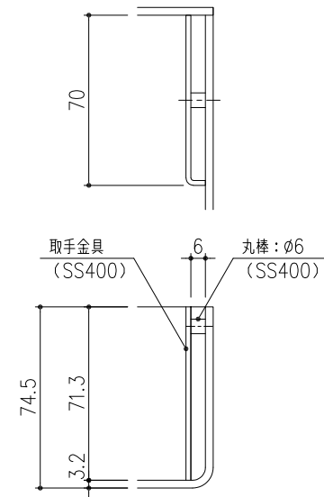
取手金具 詳細図 S=1/2
