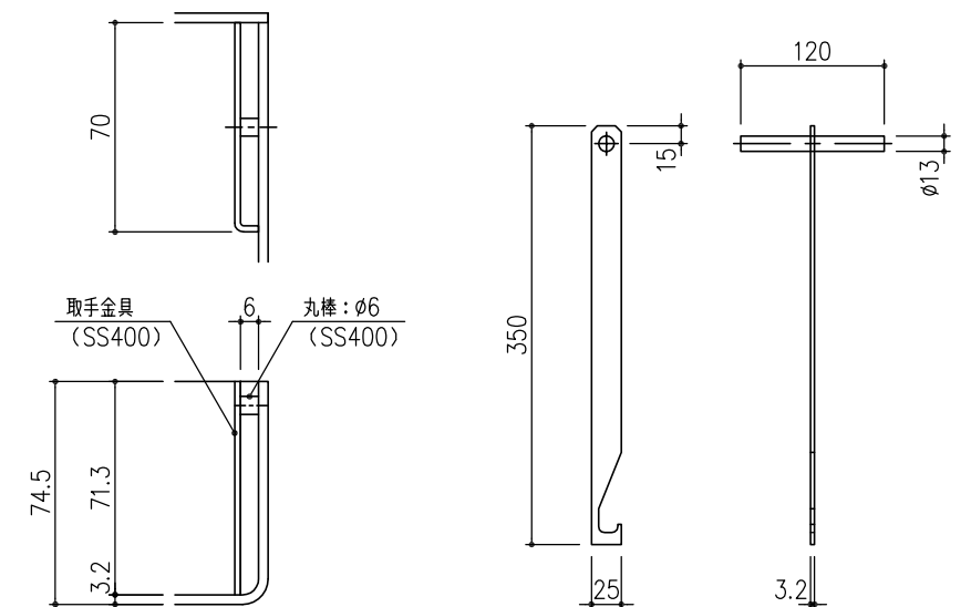
取手金具 詳細図 S=1/2
