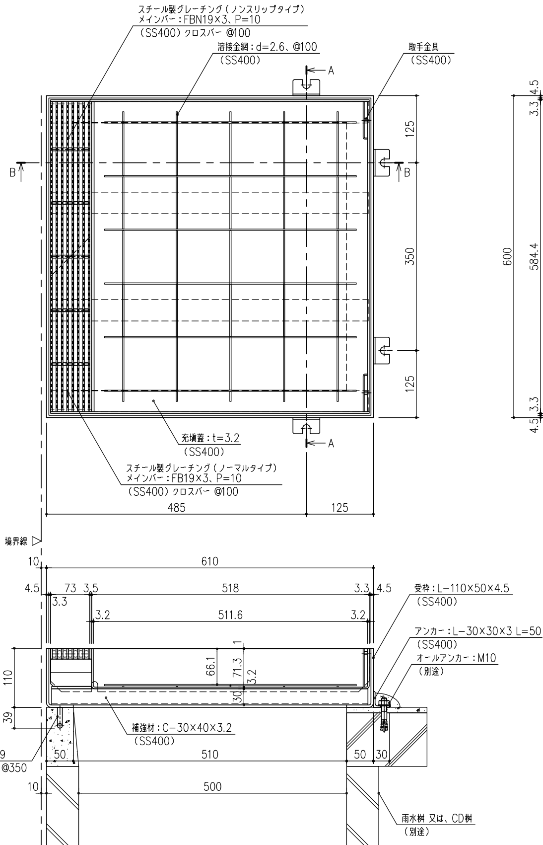
断面：B—B
