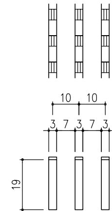
メンバー詳細図 S=1/1
