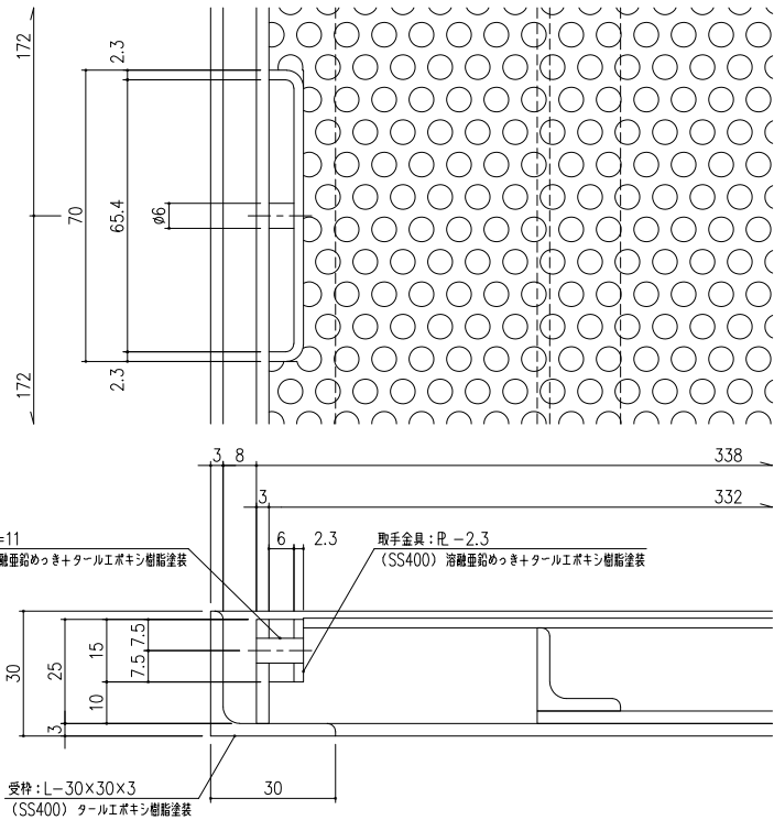
取手部 詳細図 S=1/1
