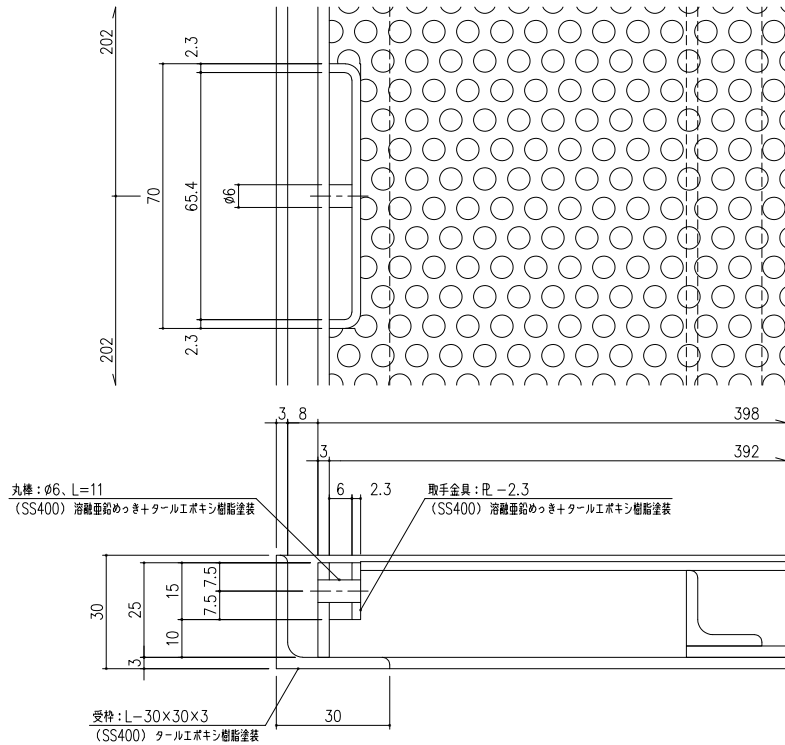
取手部 詳細図 S=1/1
