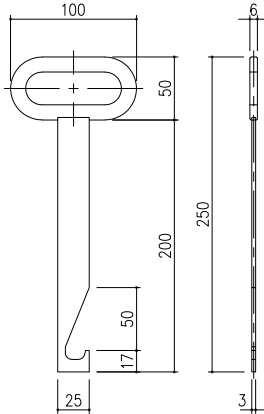
オプション: 開閉フック MF-20 (SS400) 電気亜鉛めっき
