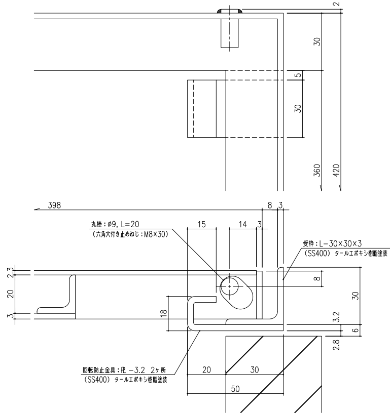
ピンジ部 詳細図 S=1/1
