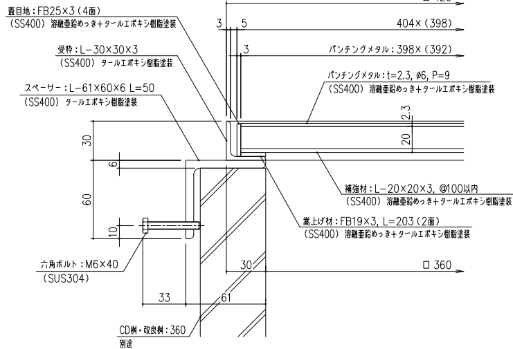
部分断面詳細図 S=1/2
