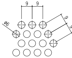
パンチングメタル 詳細図 S=1/1
