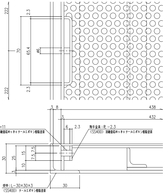
取手 部 詳細図 S=1/1
