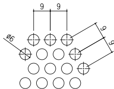
パンチングメタル 詳細図 S=1/1
