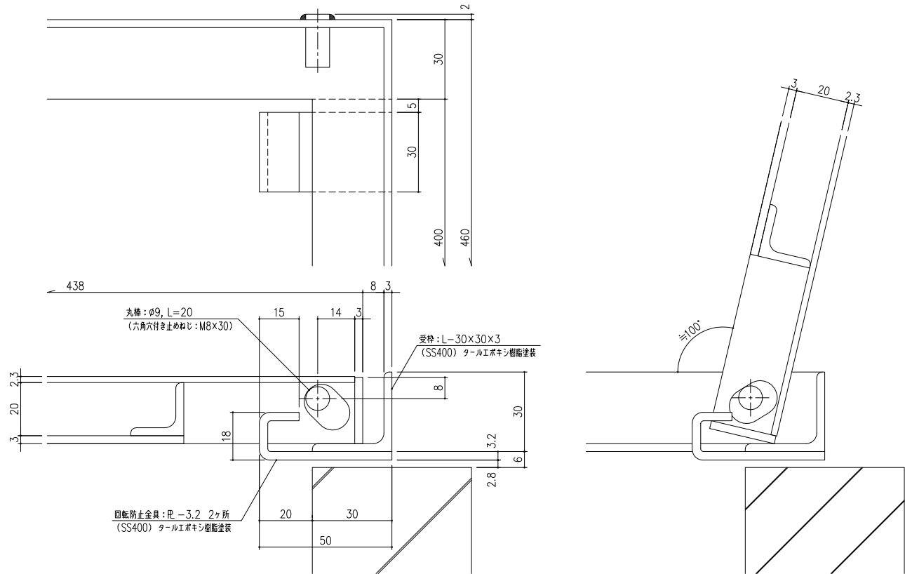
ヒンジ 部 詳細図 S=1/1
