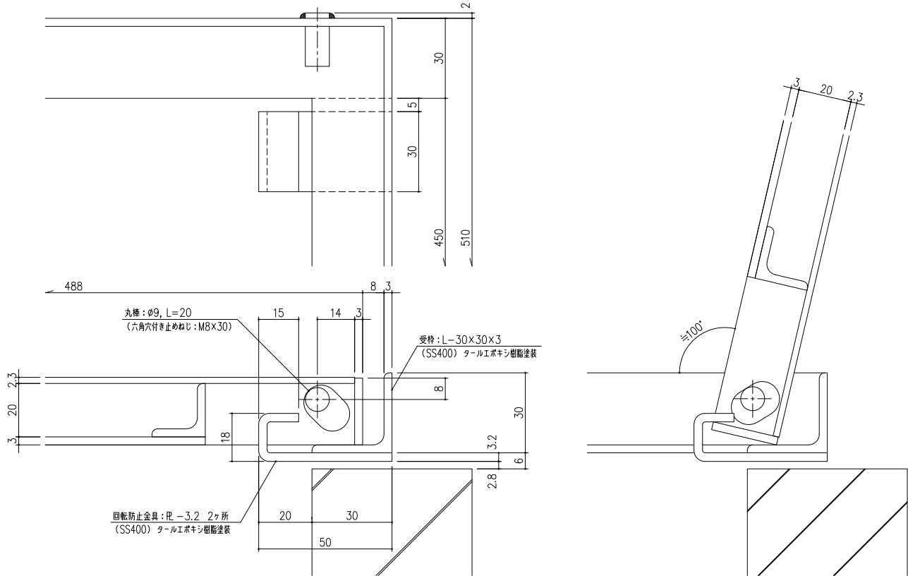
ピンジ部 詳細図 S=1/1
