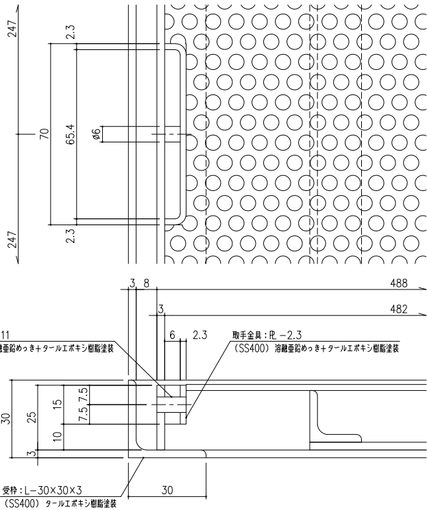
取手部 詳細図 S=1/1
