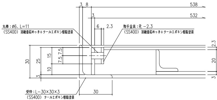
取手部 詳細図 S=1/1
