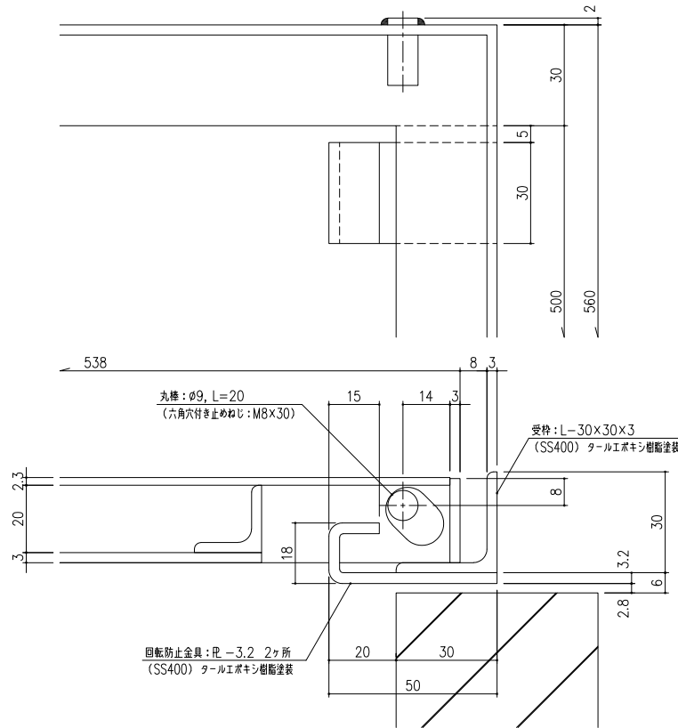
ヒンジ部 詳細図 S=1/1
