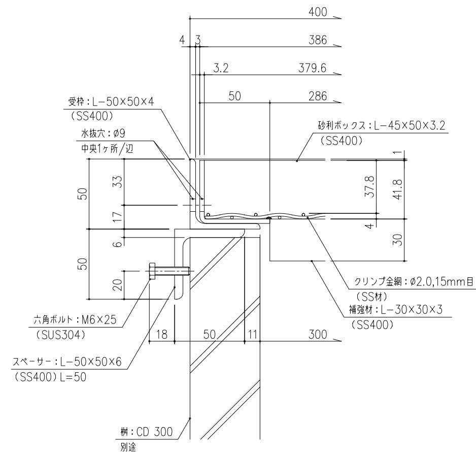
部分断面詳細図 S=1/2
