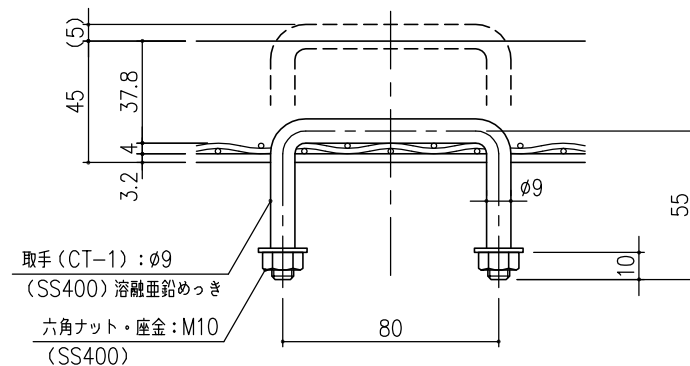
取手 詳細図 S=1/2
