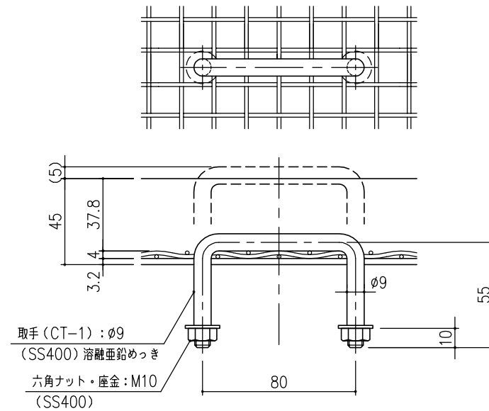
取手 詳細図 S=1/2
