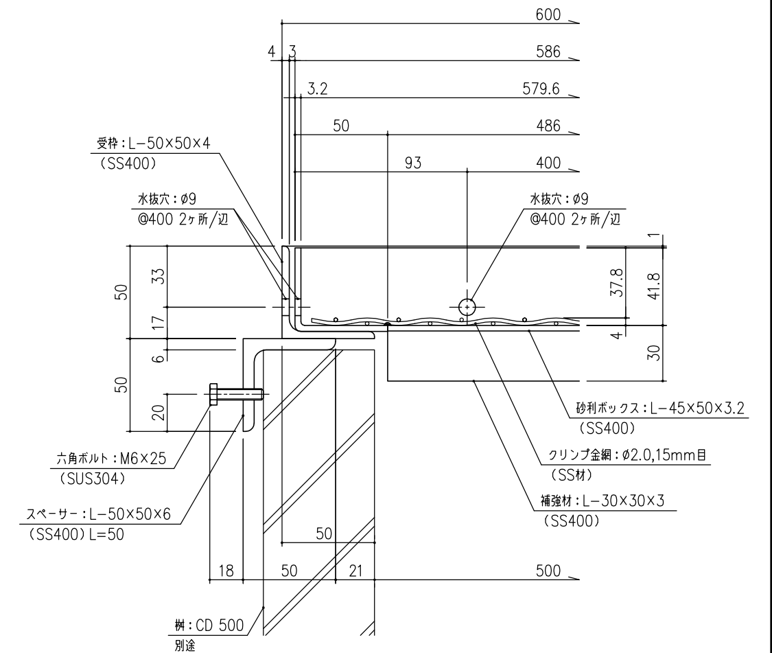
部分断面詳細図 S=1/2
