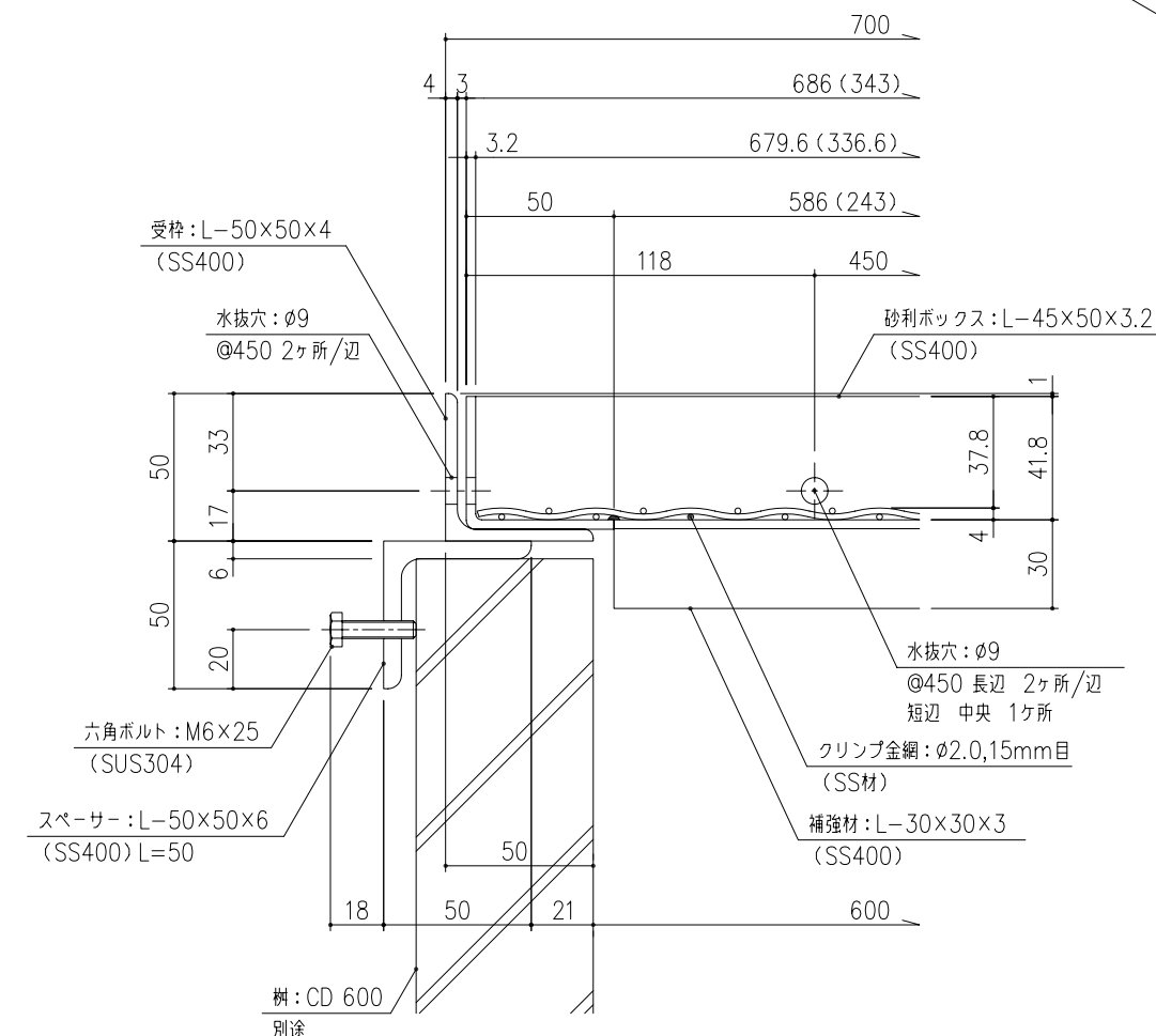
部分断面詳細図 S=1/2
