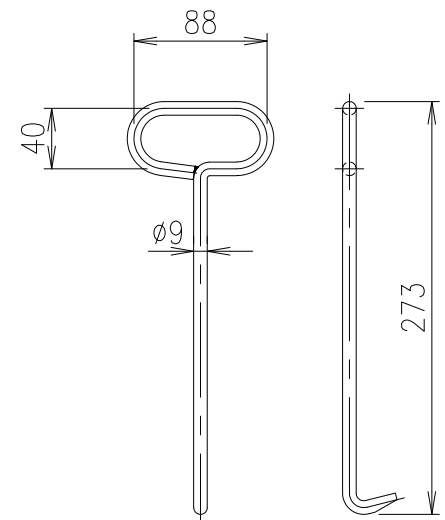
取手 (MF-1) S=1/5 (SS400) 溶融亜鉛めっき
