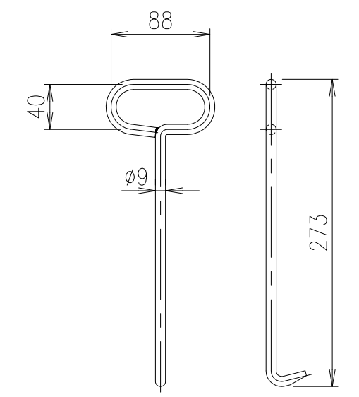
取手 (MF-1) S=1/5 (SS400) 溶融亜鉛めっき
