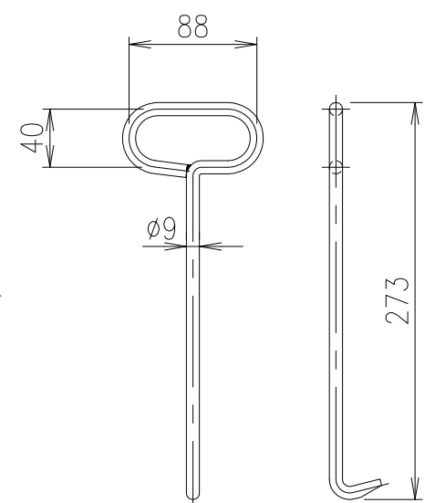
取手 (MF-1) S=1/5 (SS400) 溶融亜鉛めっき
