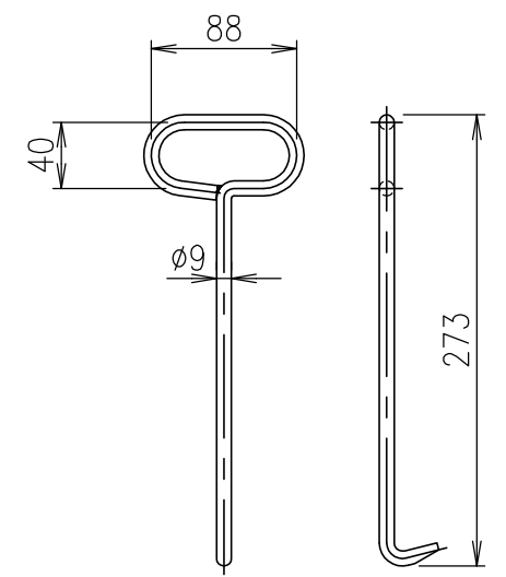
取手 (MF-1) S=1/5 (SS400) 溶融亜鉛めっき
