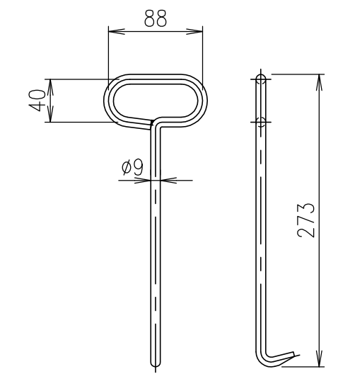
取手 (MF-1) S=1/5 (SS400) 溶融亜鉛めっき
