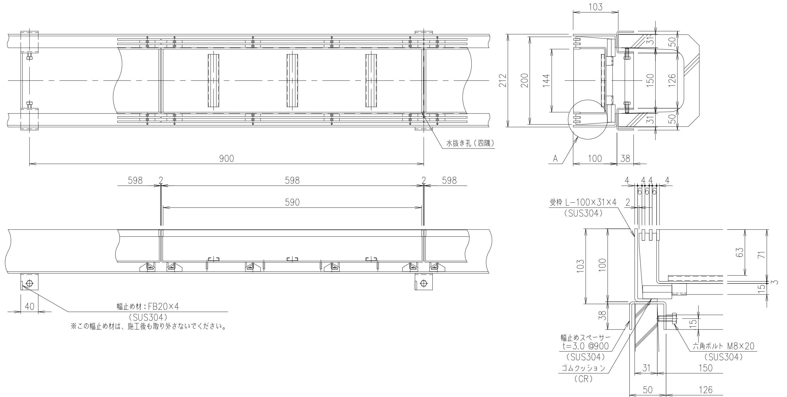
A部 詳細図 S=1/3
