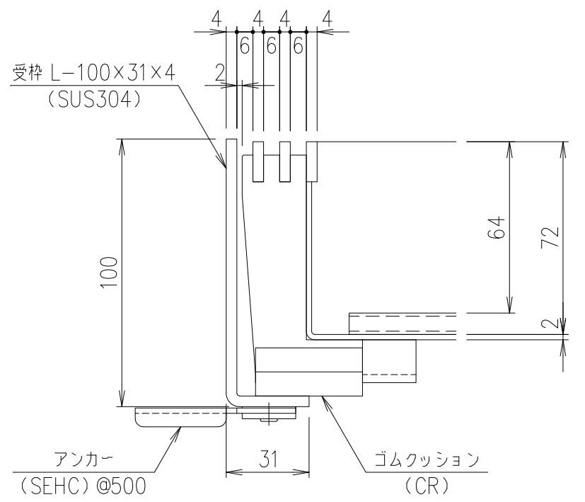
A部 詳細図 S=1/2
