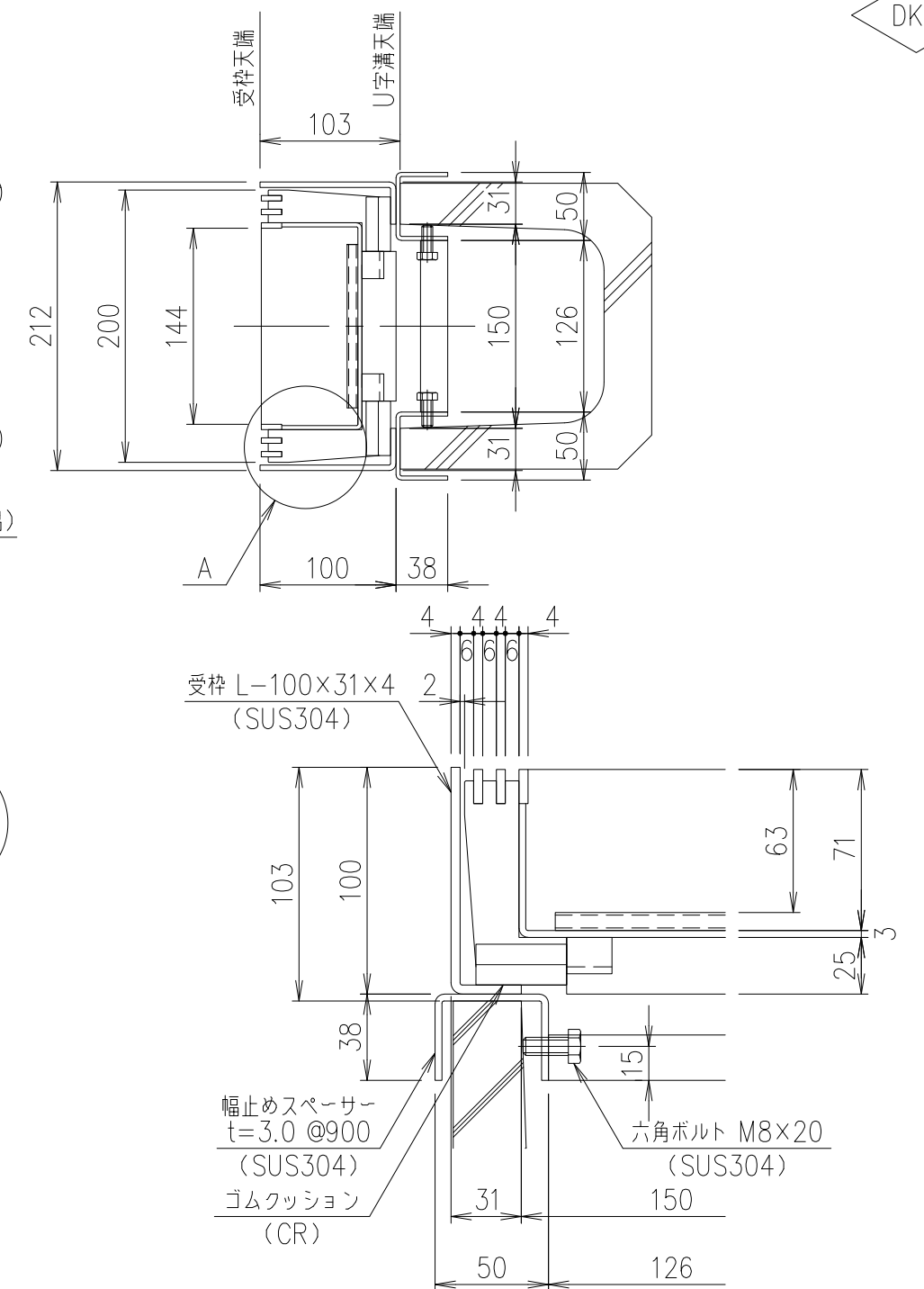
A部 詳細図 S=1/3
