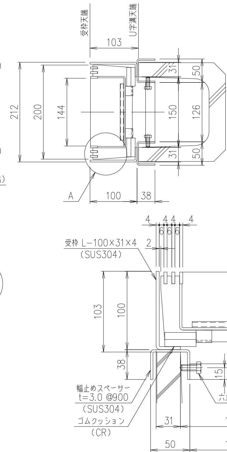
A部 詳細図 S=1/3
