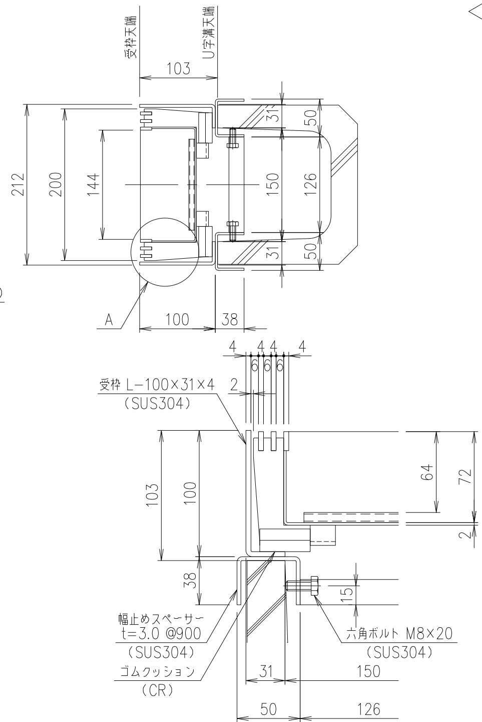
A部 詳細図 S=1/3
