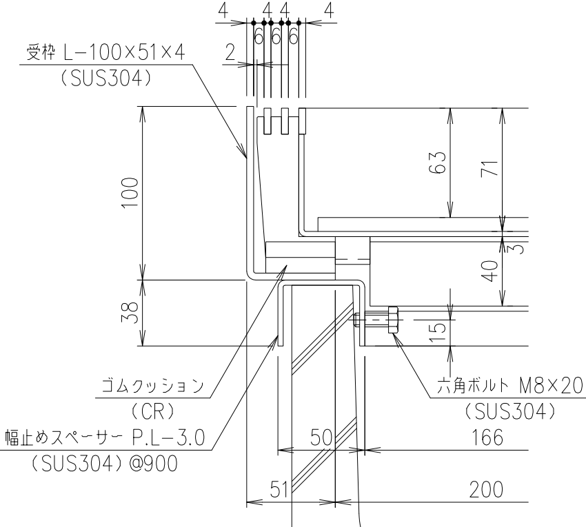
部分詳細図 S=1/3
