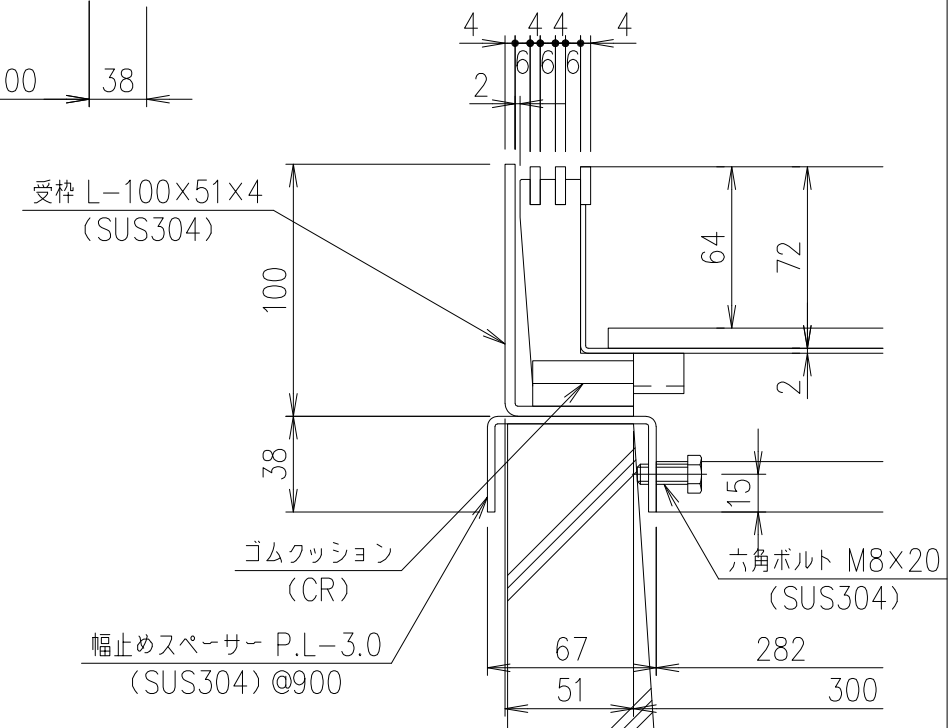
部分詳細図 S=1/3
