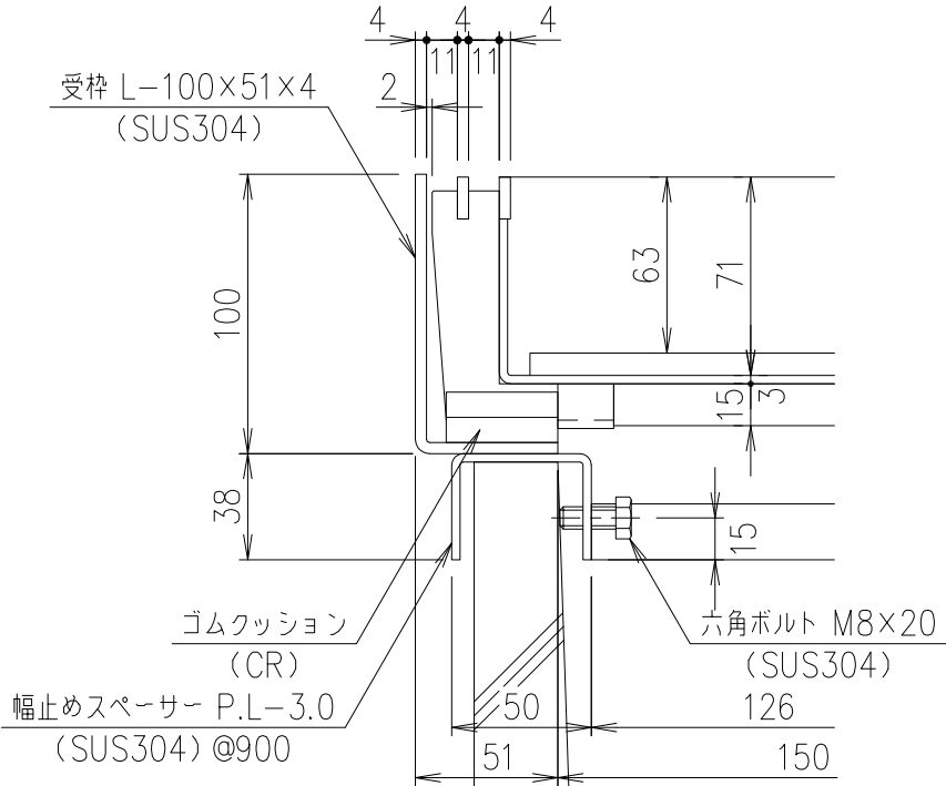
部分詳細図 S=1/3
