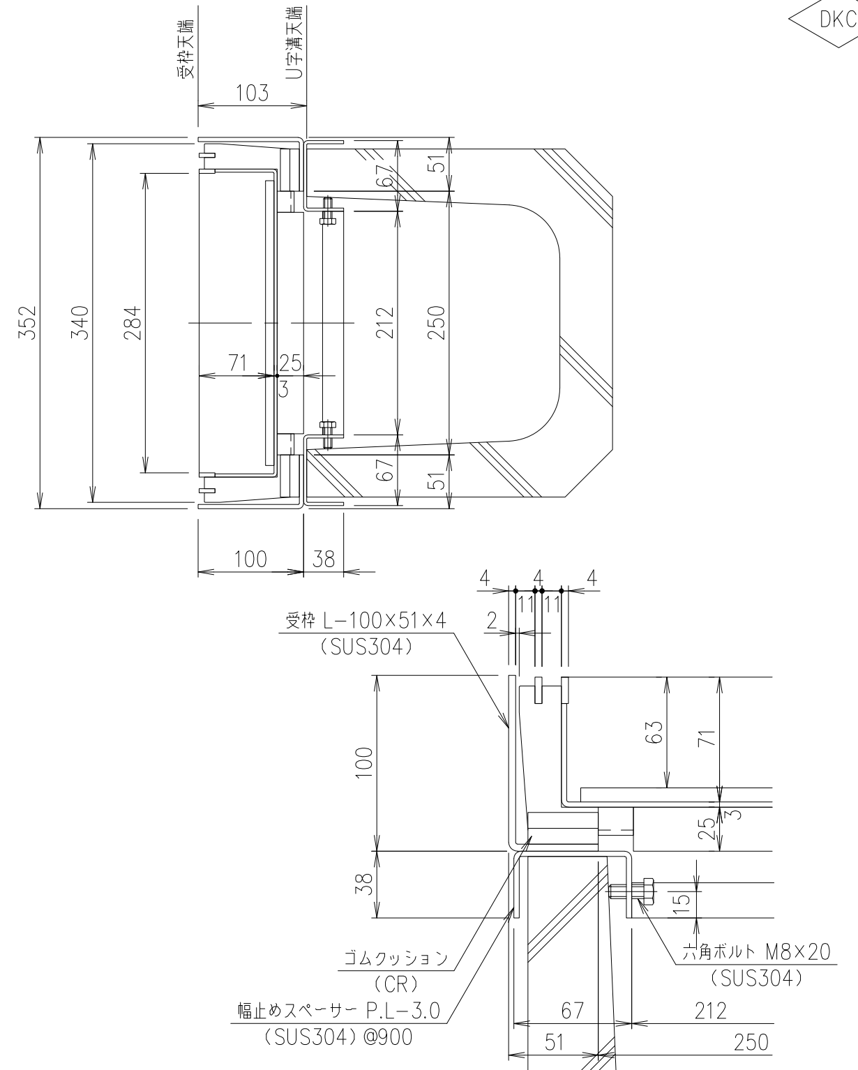
部分詳細図 S=1/3
