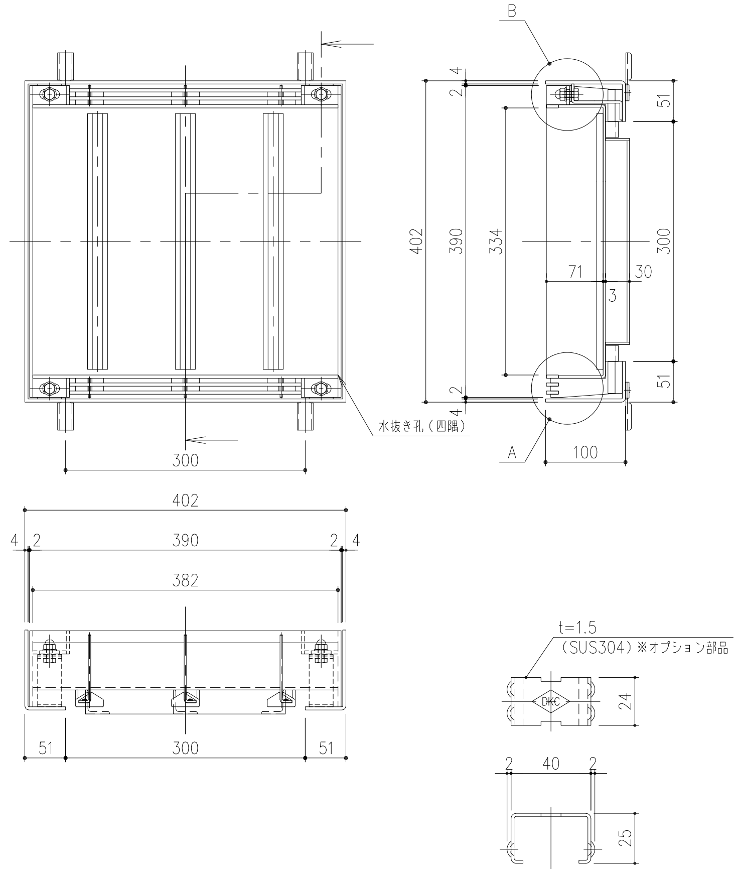
ボルト穴カバー：(特)CAP-19 詳細図 S=1/2 ※オプション部品
