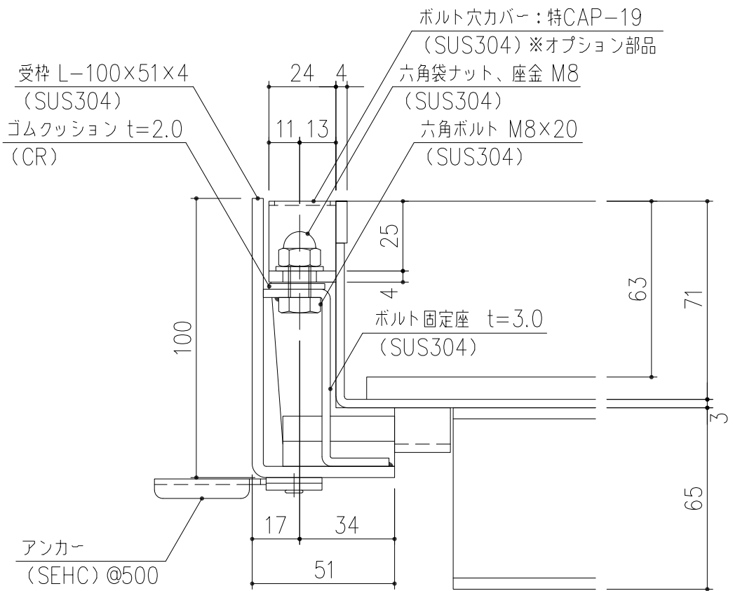
B部 詳細図 S=1/2
