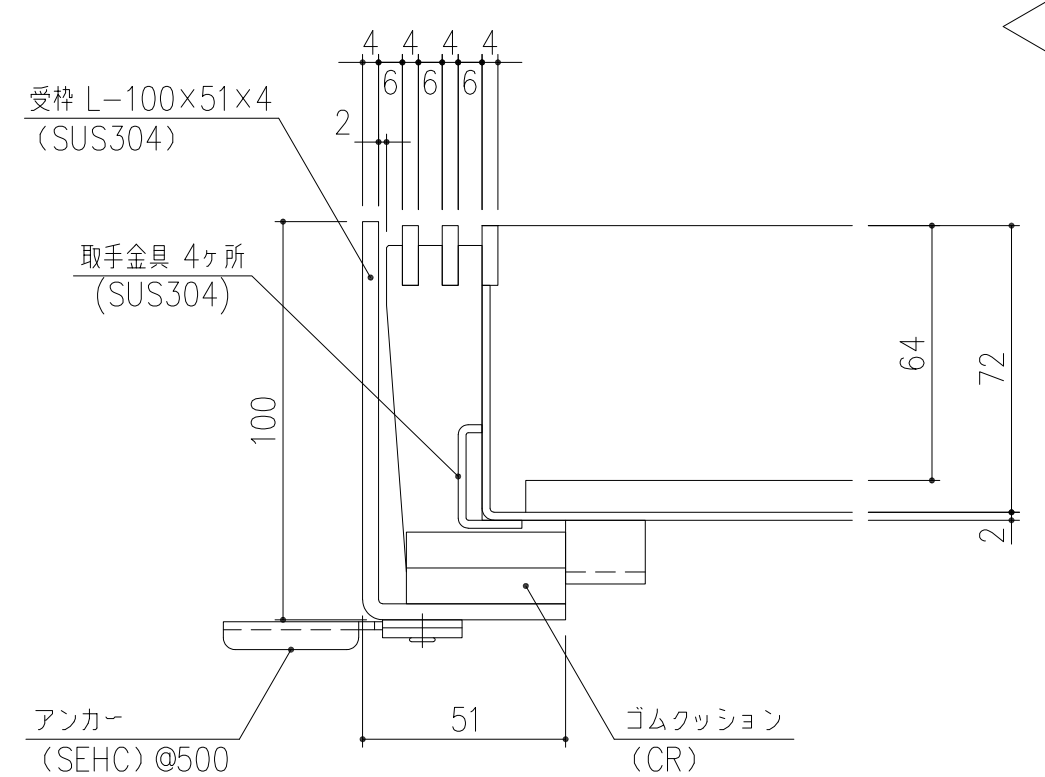
A部 詳細図 S=1/2
