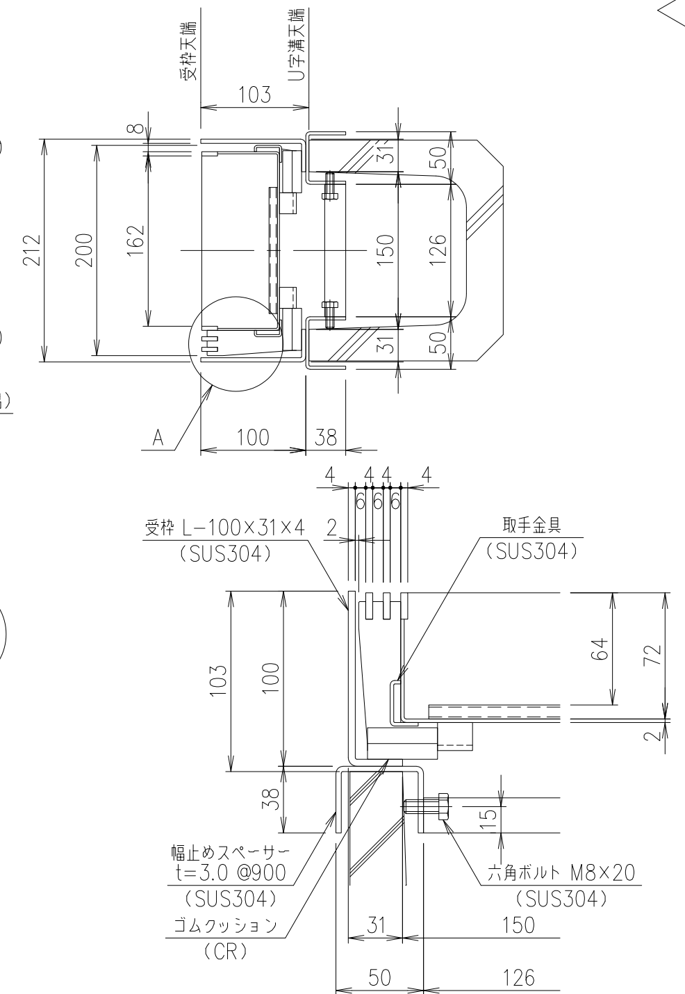
A部 詳細図 S=1/3
