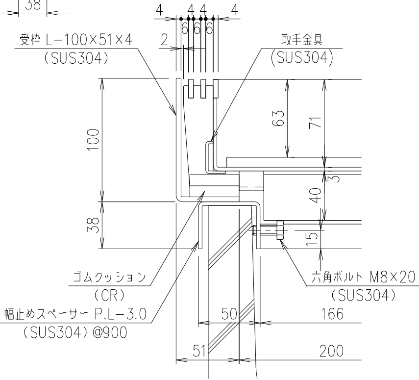
部分詳細図 S=1/3
